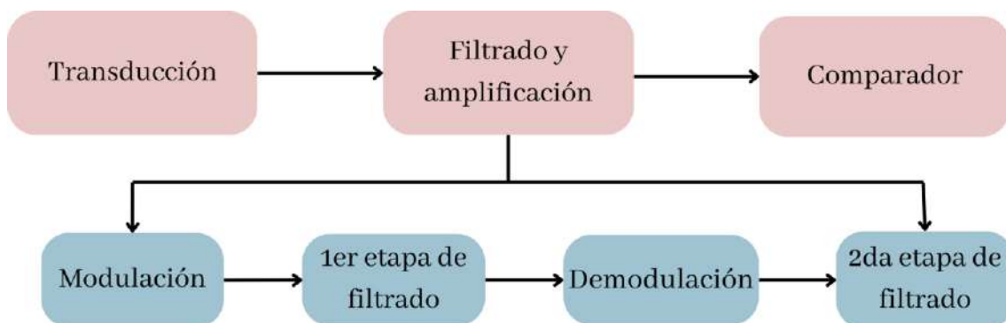
Figura 4.4 Etapas del acondicionamiento
