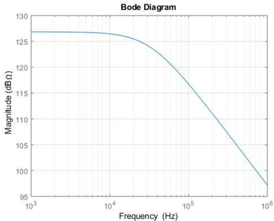
Figura 4.6 Diagrama de Bode de Amplitud
