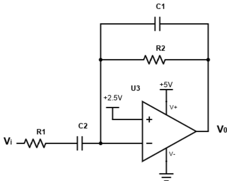
Figura 4. Filtro RC 2do orden
