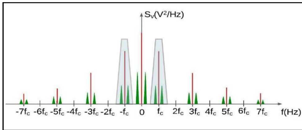
Figura 4.13 Representación en frecuencia del primer filtrado
