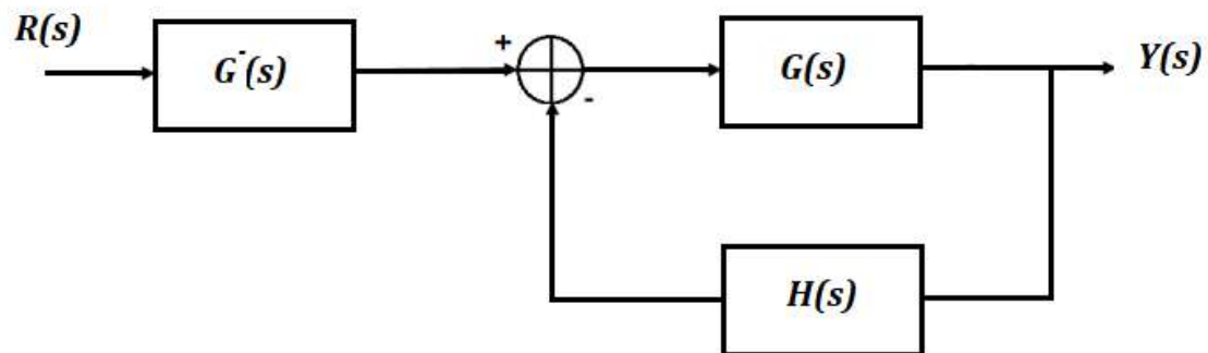
Figura 4.7 Diagrama en bloques de estabilidad
