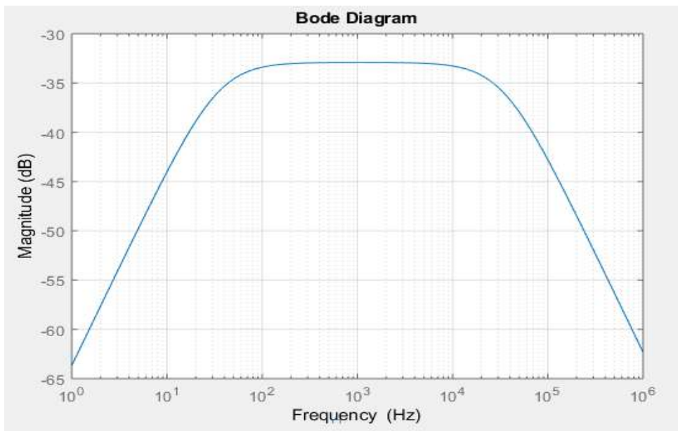
Figura 4.17 Diagrama de bode de amplitud de G^-(s)
