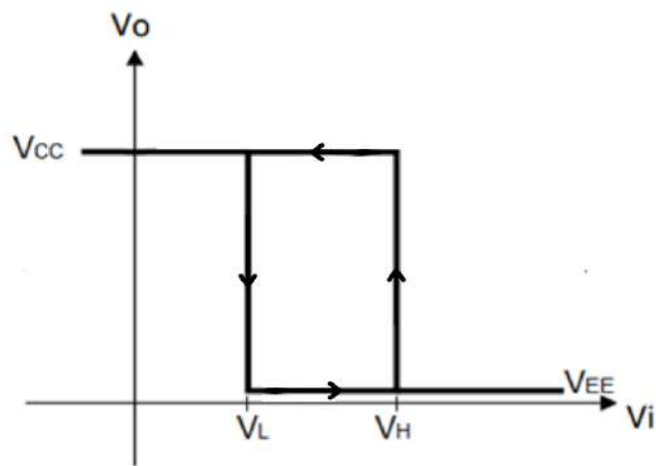
Figura 4.26 Gráfico Salida Vs Entrada comparador
