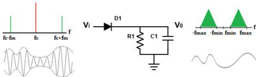
Figura 4.19 Diagrama detector de envolvente
