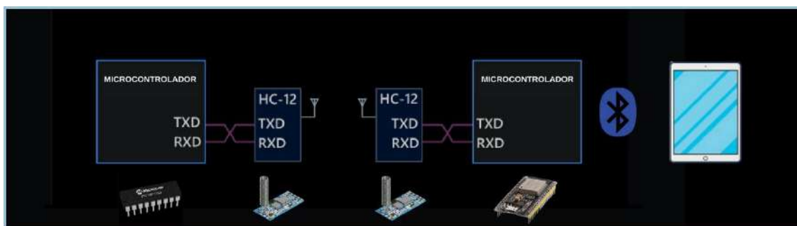
Figura 4.31 Esquemático de transmisión y recepción
