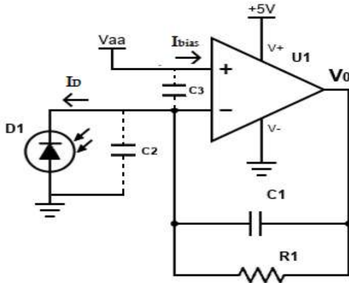
Figura 4.5 Amplificador de transimpedancia
