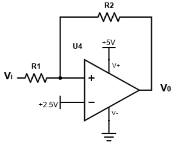
Figura 4.25 Comparador con histéresis
