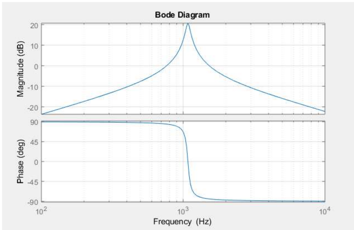
Figura 4.15 Diagrama de bode Filtro MFB
