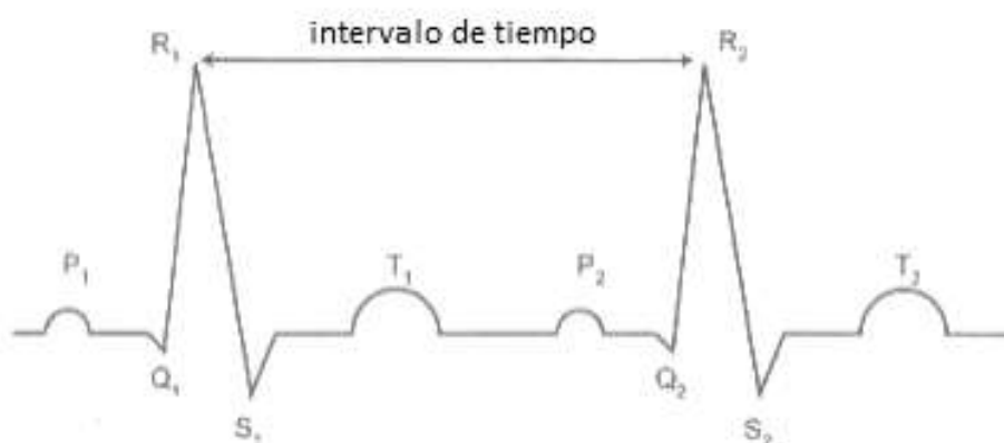
Figura 3.1 Señal ECG.
