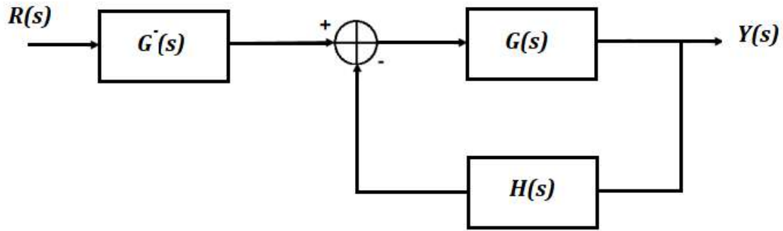
Figura 4.22 Diagrama en bloques de estabilidad
