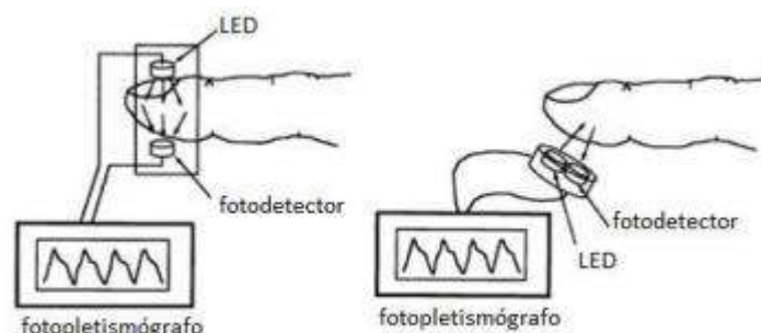
Figura 3.3 Fotopletismografía por transiluminación (izquierda) y por reflexión (derecha).
