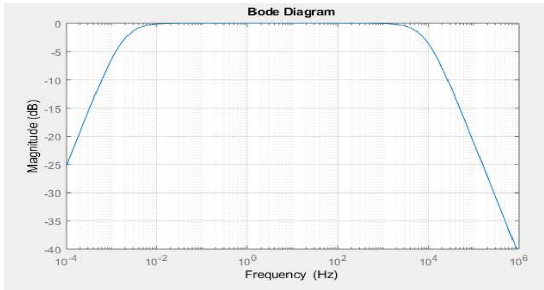
Figura 4.23 Diagrama de bode de amplitud de G^-(s)
