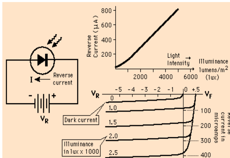
Figura 4.3 Curva característica general de un fotodiodo
