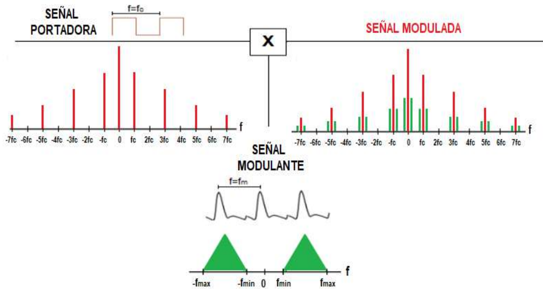
Figura 4.12 Diagrama de modulación
