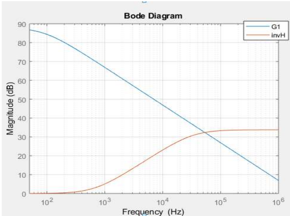
Figura 4.8 Diagrama de Bode G(s) vs 1/H(s)
