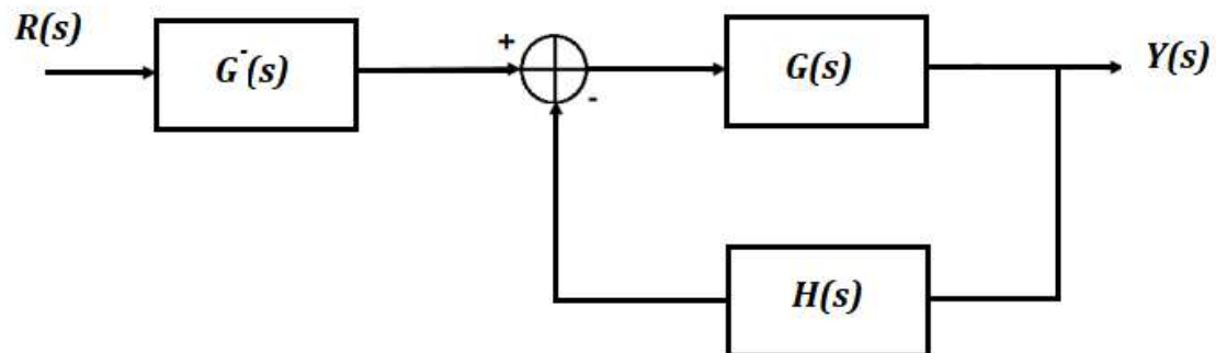
Figura 4.16 Diagrama en bloques de estabilidad
