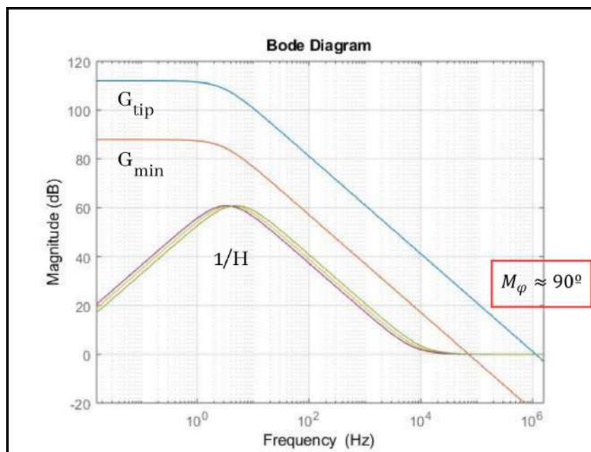
Figura 4.24 Diagrama de Bode G(s) vs 1/H(s)
