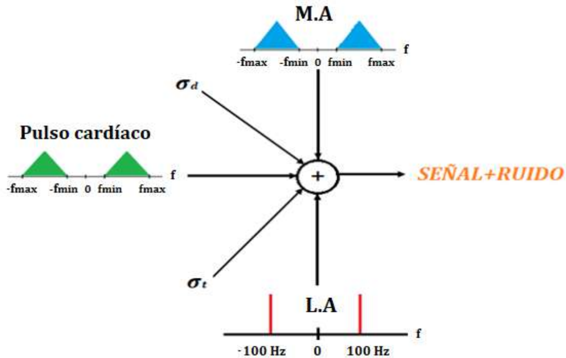
Figura 4.11 Fuentes de ruido
