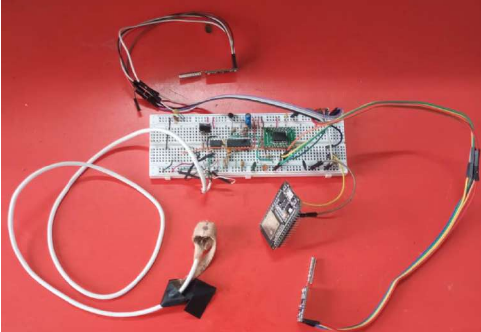
Figura 4.39 Implementación del circuito completo en protoboard
