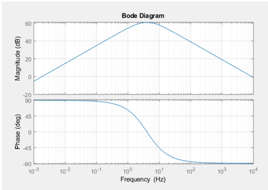
Figura 4.21 Diagrama de Bode Filtro RC 2do orden
